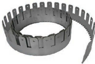
Retaining Collar - ยาว 7 m (ใช้สำหรับท่อ PVC ขนาดใหญ่กว่า 4" ขึ้นไป)
